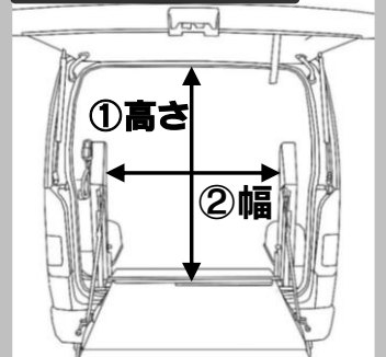
リフト取付時の有効寸法
